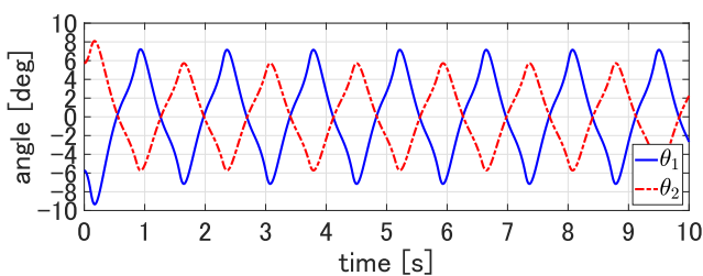
図9 不感帯を0.2の時のシミュレーションした角度
