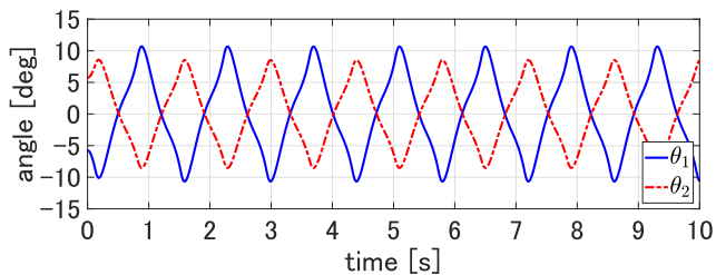
図10 不感帯を0.3の時のシミュレーションした角度
