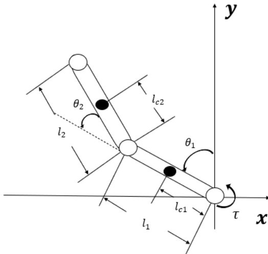
図 1 Pendubot のモデル
