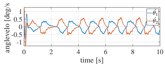
図 5 角速度 グラフ
