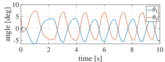
図 4 角度 グラフ
