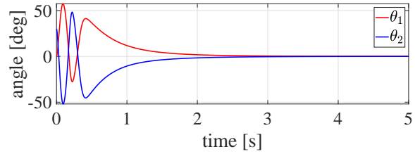
図 3 最適制御のシミュレーション
