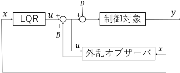
図 12 外乱オブザーバの構成
