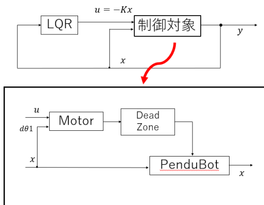
図7 摩擦を考慮したPendubot実験機の構図
