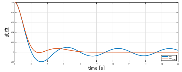
図 13 外乱オブザーバによる補償を行っていない場合と行った場合の比較結果
