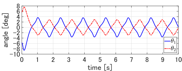
図8 不感帯を0.1の時のシミュレーションした角度
