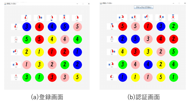
図3 実装画面
